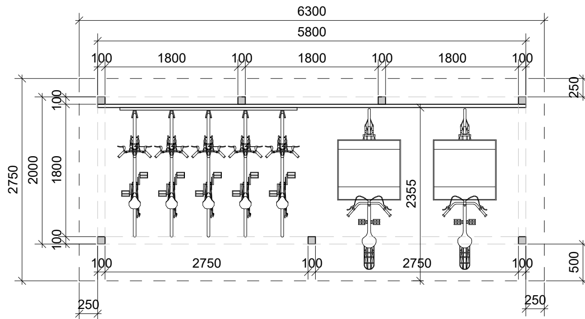
FAST cykeloverdækning med plads til én række cykler. Kan forlænges med elementer af 1.800 mm/stk.
