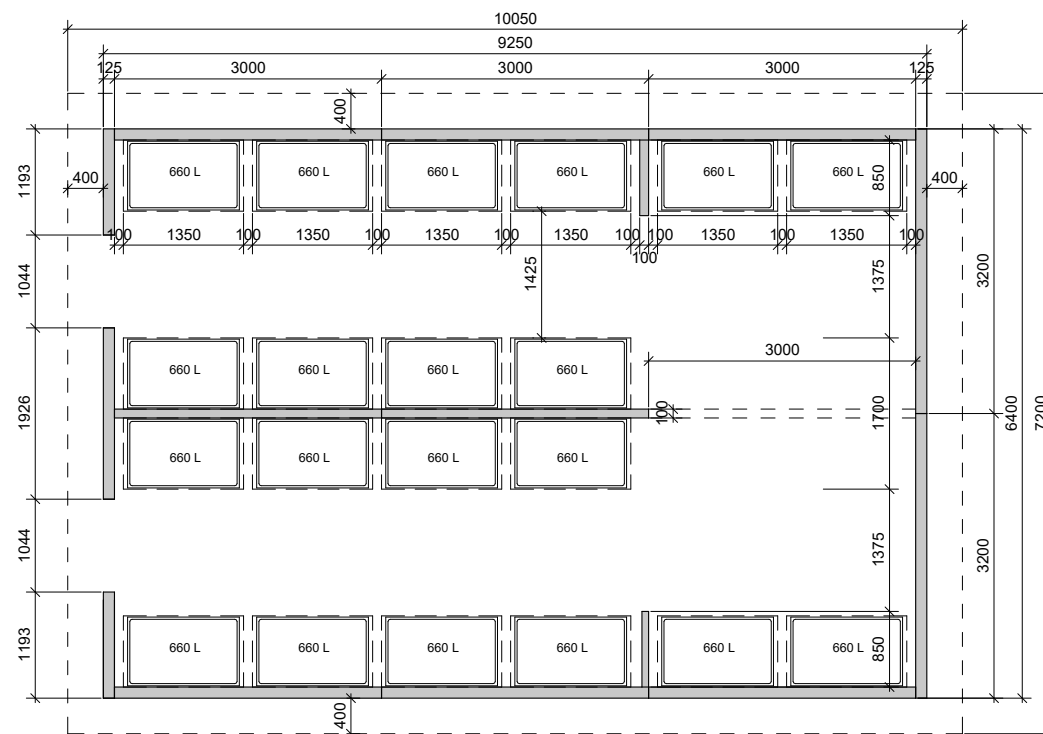
FAST affaldsskur med plads til 4 rækker affaldscontainere - kan forlænges med elementer af 3000 mm.
